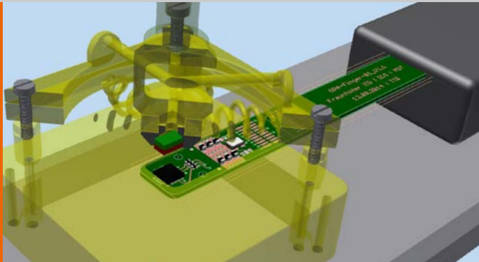
Prototyp eines 6D-Messsystems:
